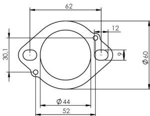
S.S. Flange 112A P/N 204569R sp. 5mm
